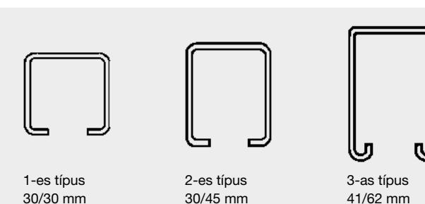
12. ábra: Profilsíntípusok
