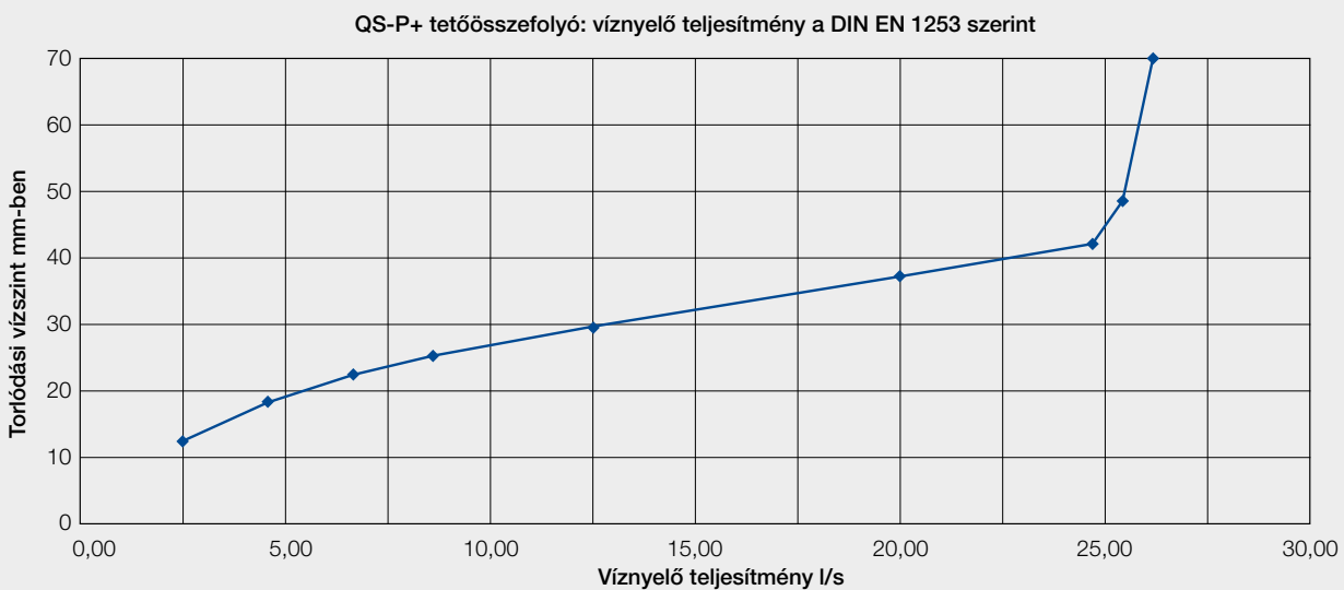
41. ábra: QS-P+ víznyelési teljesítmény grafikon (a DIN EN 1253-2 szerint)
