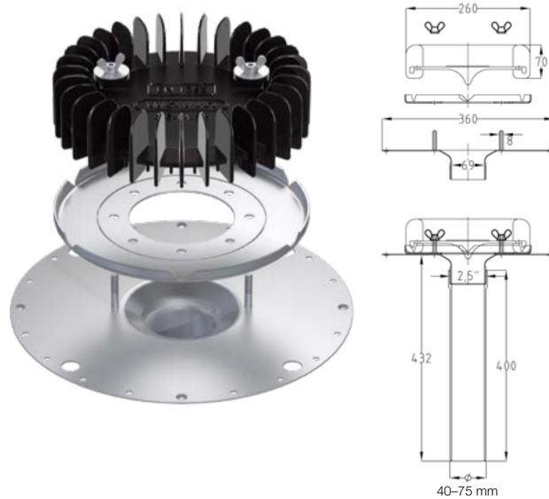
QS-M-75-260 tetőösszefolyó víznyelő teljesítménye
