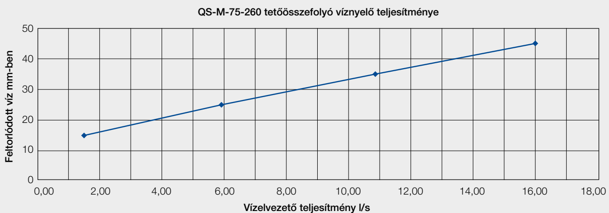
43. ábra: Víznyelési teljesítmény grafikon QS-M-75-260 tetőösszefolyóhoz
