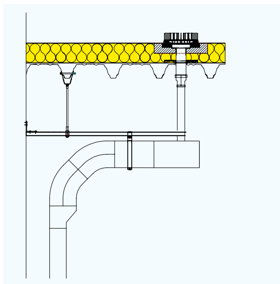
10. ábra: Szűkített ejtővezeték
