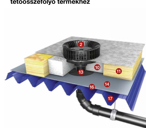
38. ábra: QS-P+ meleg tetős vízelvezető alaprendszer
