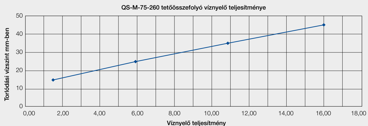
44. ábra: QS-M-75-260 tetőösszefolyó víznyelési teljesítmény grafikonja, (DIN EN 1253)
